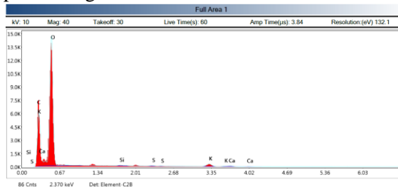
Gambar-17. Visualisasi hasil SEM untuk Buah Pada Gambar-17. hasil SEM tidak terdapat logam berat yang berada di menempel pada buah tanaman cabai rawit.
