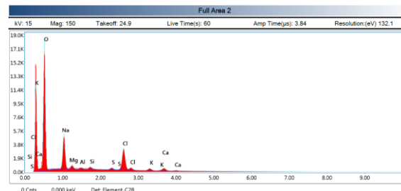
Gambar-7. Visualisasi hasil SEM untuk Daun
