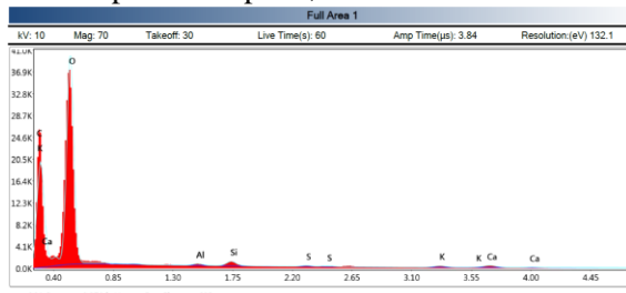
Gambar-13. Visualisasi hasil SEM untuk Batang Pada Gambar-13. hasil SEM tidak terdapat logam berat yang berada di menempel pada batang tanaman.
